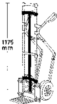
Hulpstuk Type 1190 Middenstrip, alu. t.b.v. alu. steekwa- gens 1300 mm hoog met 2 extra kunststof dwarsverbindingen
