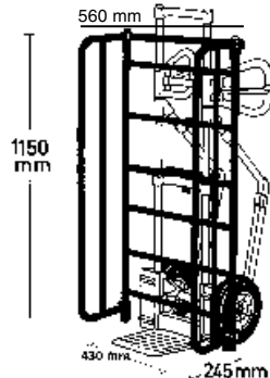
Hulpstuk Type 1311 Laadvlakverbreding-rek voor alu. steekwagens, zijden inklapbaar
