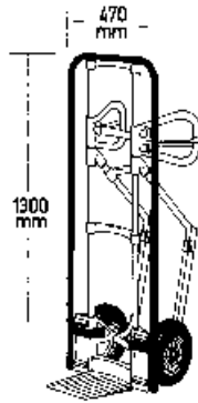
Hulpstuk Type 1197N Holmverbreding aanlegvlak
