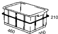
kunststof krat met houder Type 1038
