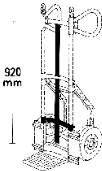
Hulpstuk Type 1196 Middenstrip, alu. t.b.v. alu. steekwagens 1100 mm hoog
