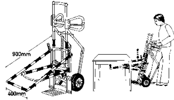
Hulpstuk Type 1050 + 1044 in hoogte verstelbare laadbeugel voor het transport van stoelen en tafels. Snel afneembaar.
