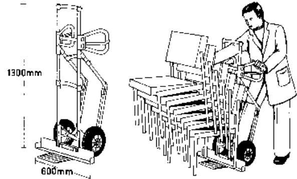
Hulpstuk Type 1029A Schopopzetstuk, aluminium, voor stoeltransport
