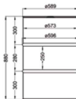
Standaard metalen vat (DS/EN 210).
