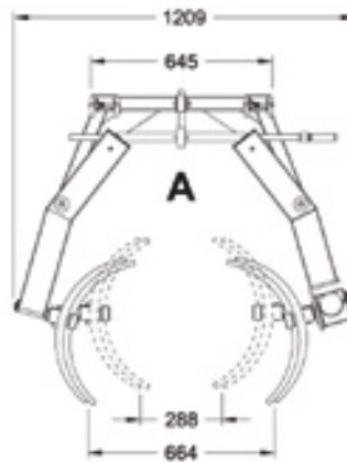
A: Vatenkantelaar voor standaard metalen vaten (DS/EN 210).
