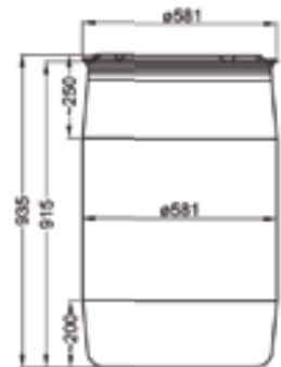
Standaard plasticen vat (DS/EN 12707).
