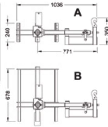
B: Vatenkantelaar voor standaard plasticen vaten (DS/EN 12707).
