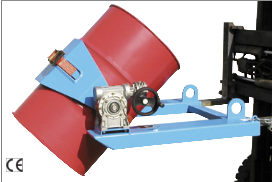
Type 565.FLEX-HK, lediging van 200 liter stalen stopvat
